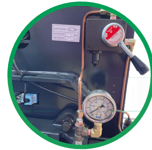
HYDRAULISCHE BANDSPANINRICHTING
